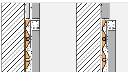
Wariant montażowy: ścienny profil ograniczający Schlüter®-QUADEC
