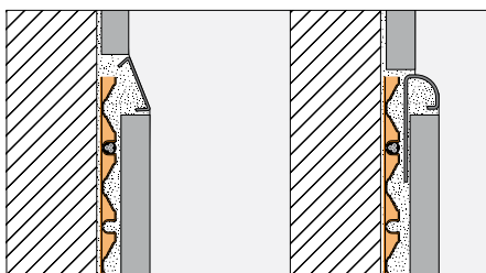
Warianty montażowe: ścienne profile ograniczające Schlüter®-DESIGNLINE Schlüter®-RONDEC
